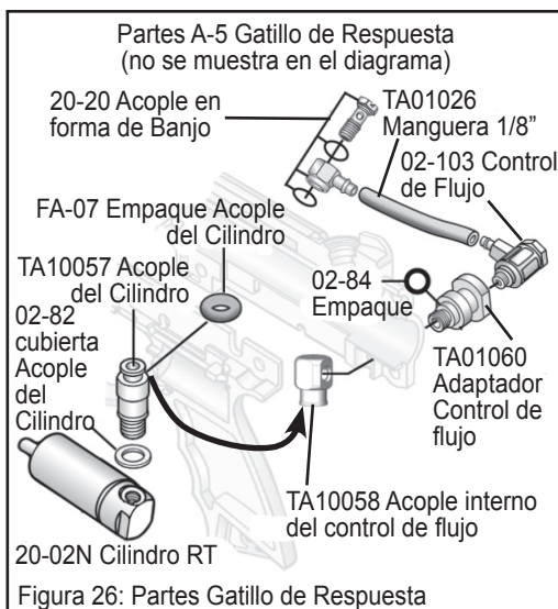
Figura 26: Partes Gatillo de Respuesta
