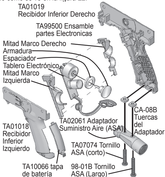
Figura 21: Diagrama Partes internas E-Grip
