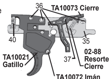
Figura 19: Ensamble Gatillo E-Grip
