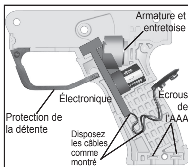
Figure 22: Électronique du récepteur inférieur
