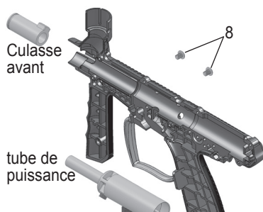
Figure 13: Enlevez le tube de puissance
