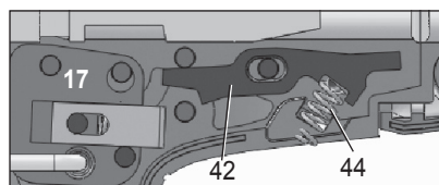
Figure 10: Emplacement de l'adaptateur de la détente, de la gâchette et du ressort de la gâchette
